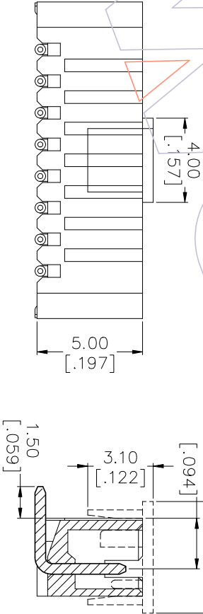
SECTION:A-A
