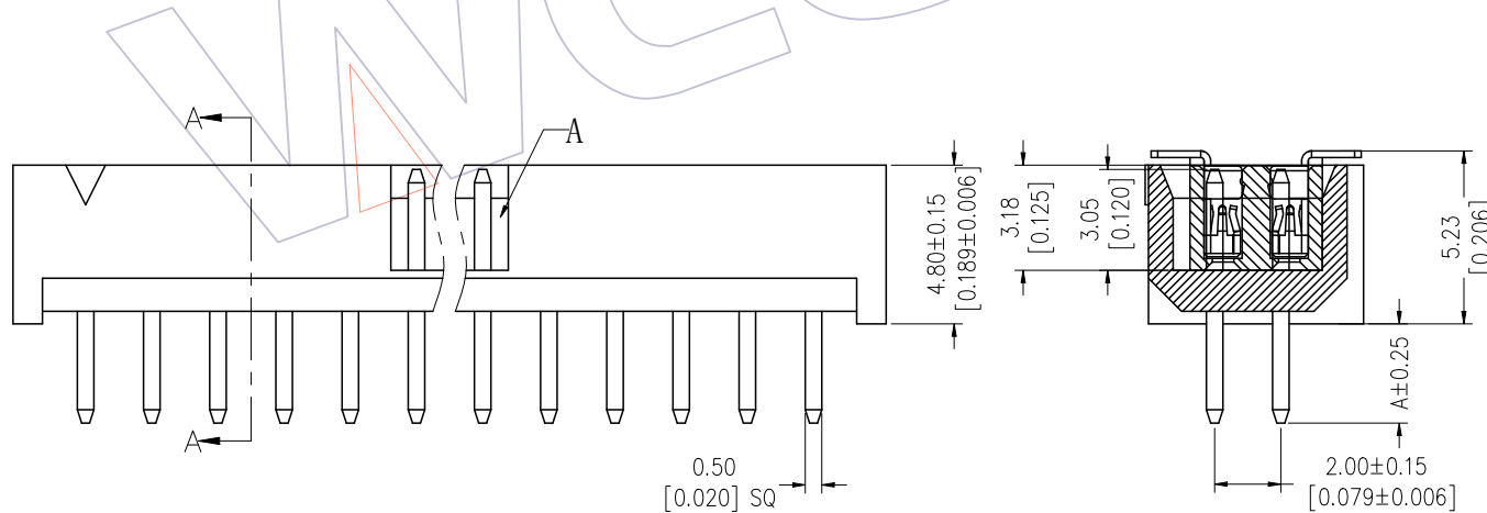
SECTION A-A
